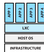
LXC Containerisation
